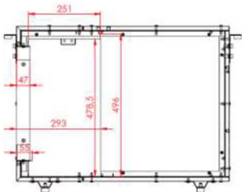
REZ A-A
