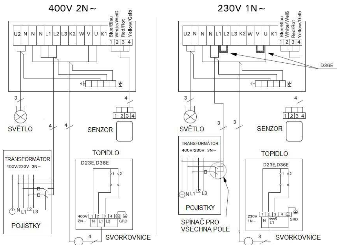
Obr. 12 Elektrické zapojení kamen (D23E, D36E) a řídící jednotky C90
