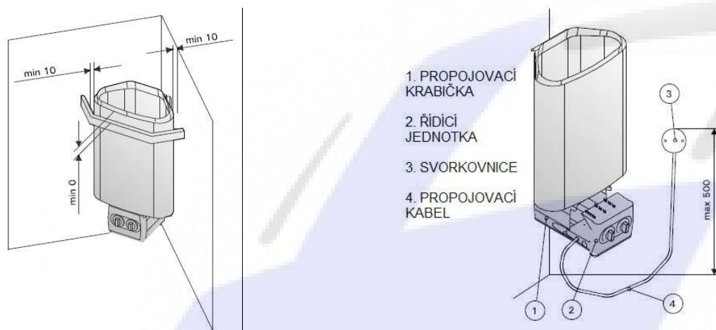
Obr. 8 Bezpečnostní ohrádka kamen Obr. 9 Elektrické zapojení kamen
