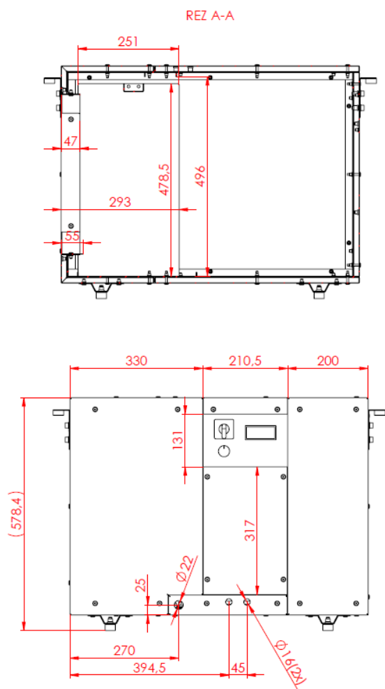
Boční pohled
