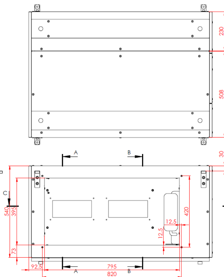
Horní pohled
