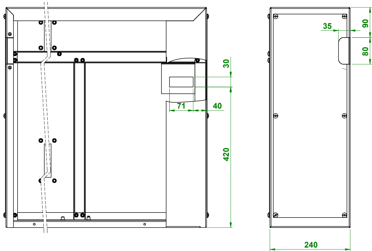
boční pohled s teplovodní vložkou
