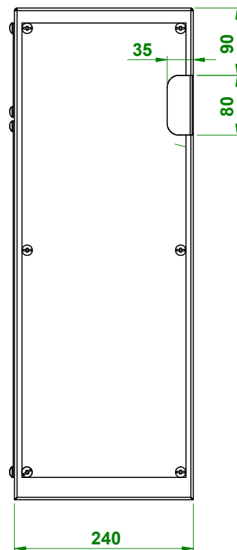
boční pohled s teplovodní vložkou
