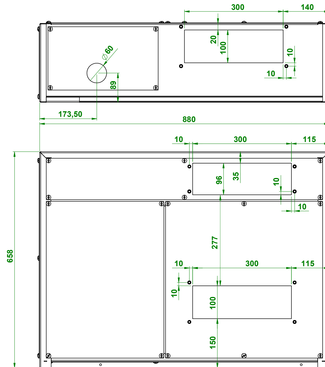
spodní pohled
