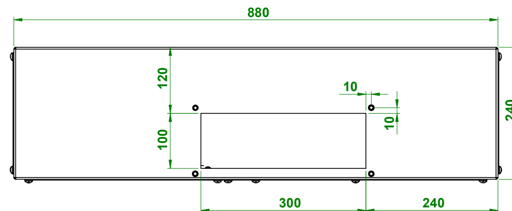
horní pohled
