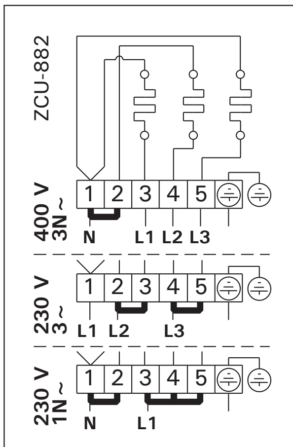
Figura 14. Conexiones eléctricas (1-E, 2-E)
