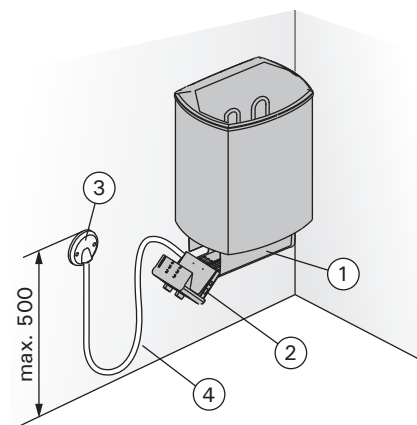
Obrázok 9. Umiestnenie montážneho nosníka ohrievača (všetky rozmery sú v milimetroch)
