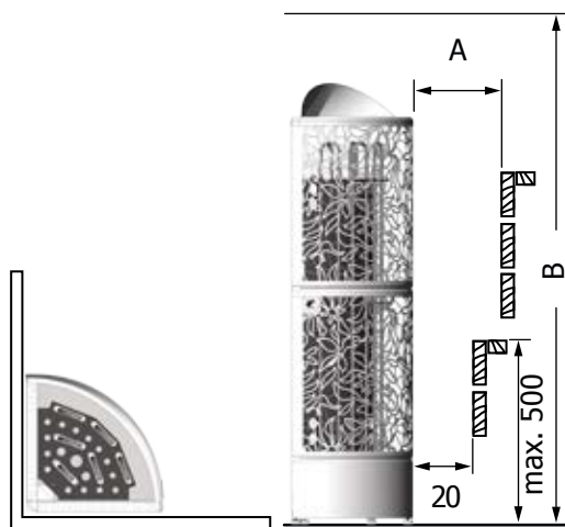
Kuva 2 | Vähimmäisetäisyydet (mm) Fig. 2 | Minimum safety distances (mm)
