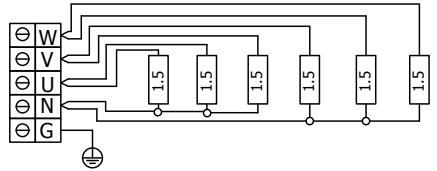
DRFT6-90NS-CNR 9,0 kW
