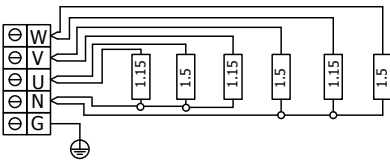
DRFT6-80NS-CNR 8,0 kW
