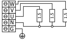
DRFT3-45NS-CNR 4,5 kW
